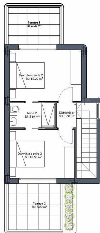
PLANTA PRIMERA
