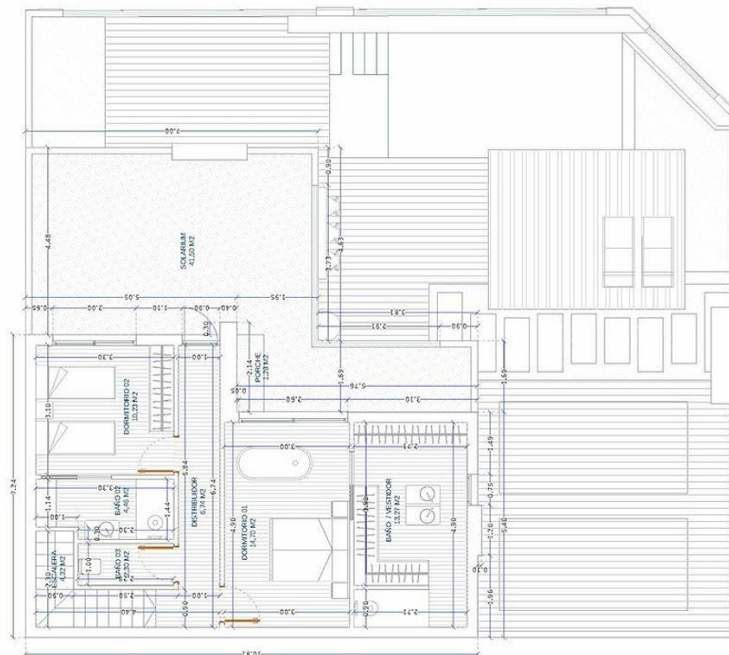
S. CONSTRUIDA VIVIENDA P.1 | 67.57 M2
