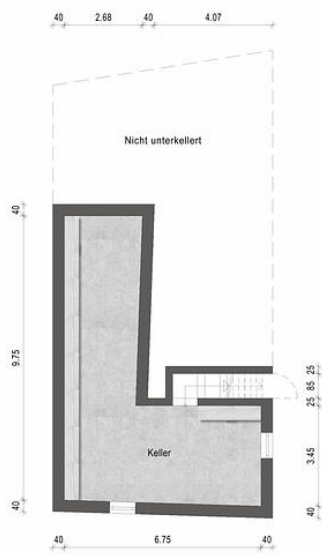
Kellergeschoss
