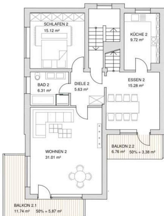
OBERGESCHOSS M=1/100
