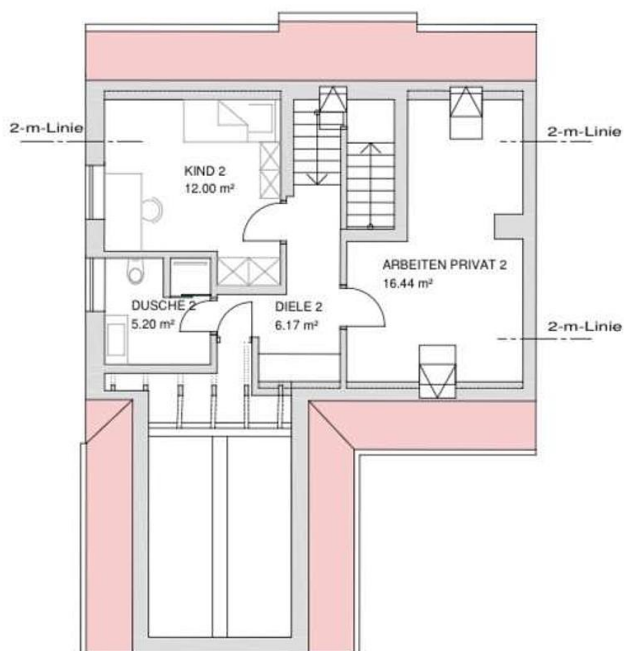
DACHGESCHOSS M=1/100
