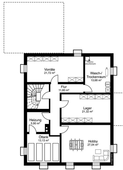
Kellergeschoss
