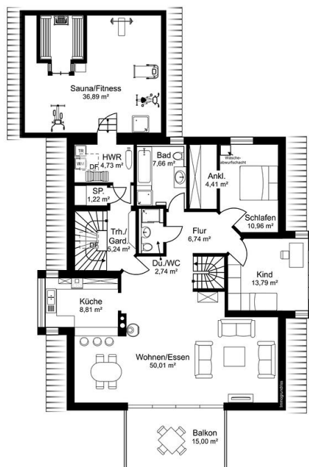
Dachgeschoss
