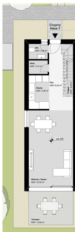
Haus 1 Erdgeschoss
