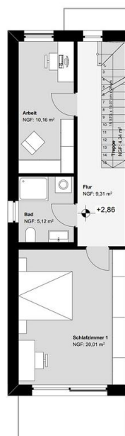
Haus 1 1.Obergeschoss
