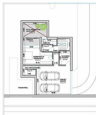
PLANTA SÓTANO / BASEMENT
