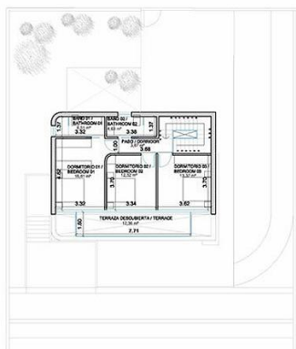
PLANTA PRIMERA / FIRST FLOOR
