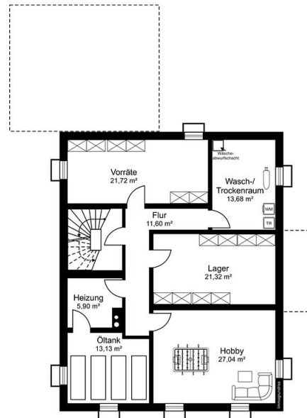
Kellergeschoss
