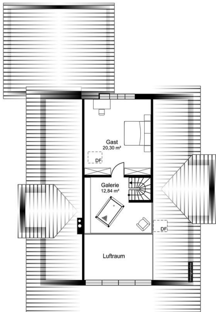
Galeriegeschoss
