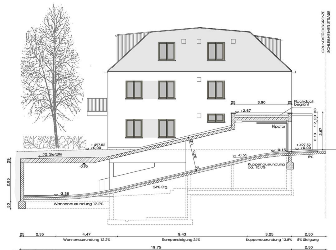
SCHNITT B-B
