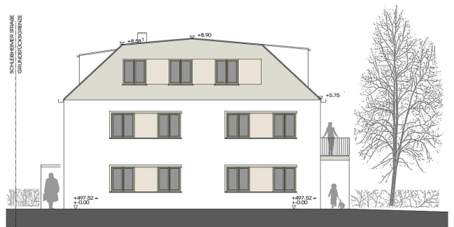
ANSICHT NORD
