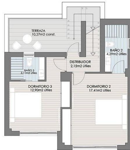
PLANTA PRIMERA E: 1/75
